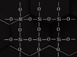
二酸化ケイ素 構造式
