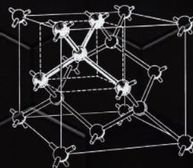
最外殻電子が4つのケイ素で形成された結晶構造。
